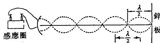
圖(六) 駐波的形成
